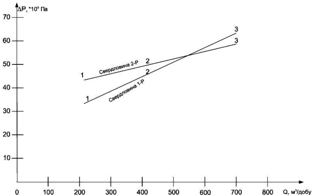
Рисунок 1 – Криві прийомистості \Delta P=f(Q)
