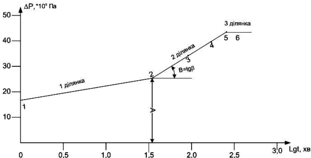
Рисунок 2 – Графік часового простежування підвищення тиску під час пробного закачування розсолу у свердловину 2-Р
