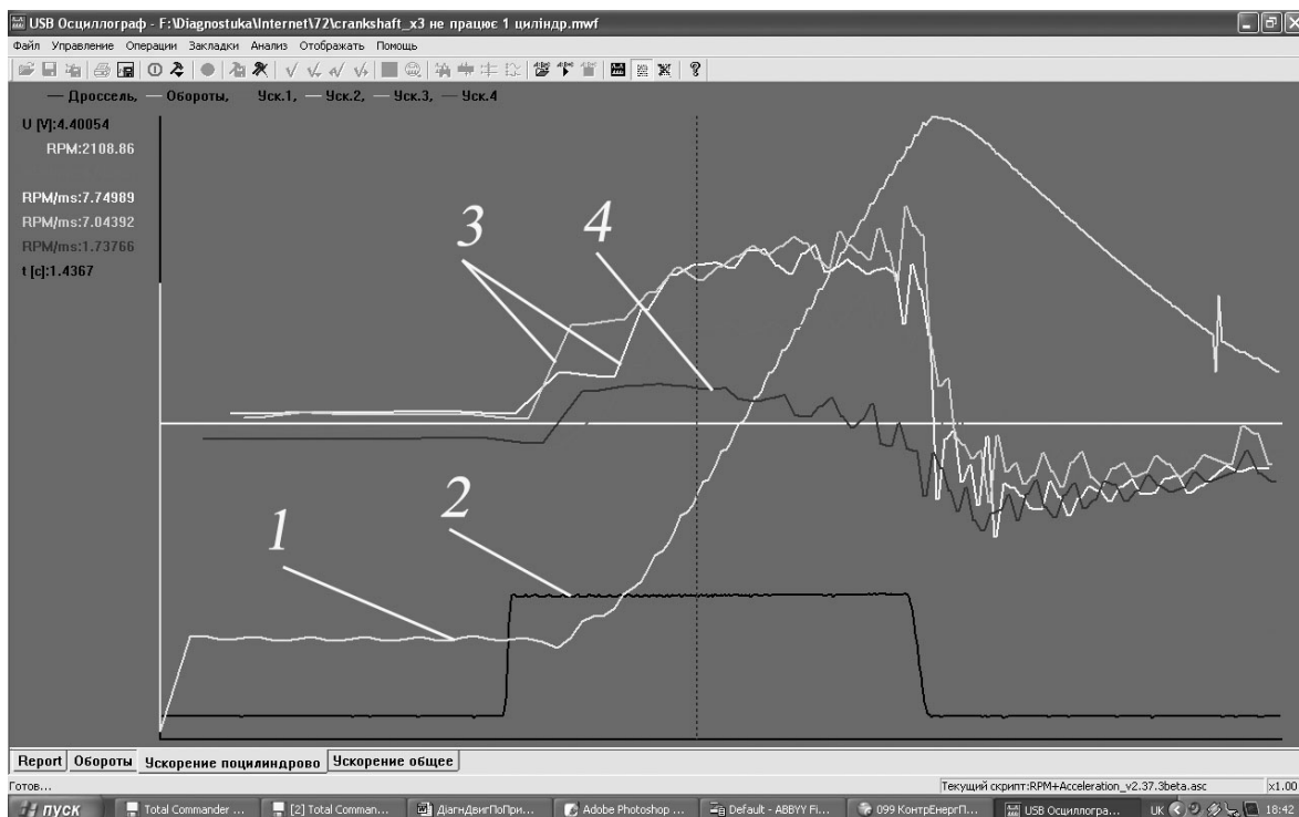
1 – сигнал частоти обертання колінчастого вала; 2 – сигнал відкриття дросельної заслінки; 3 – сигнали прискорень окремих справних цилиндрів; 4 – сигнал прискорення непрацюючого цилиндра
