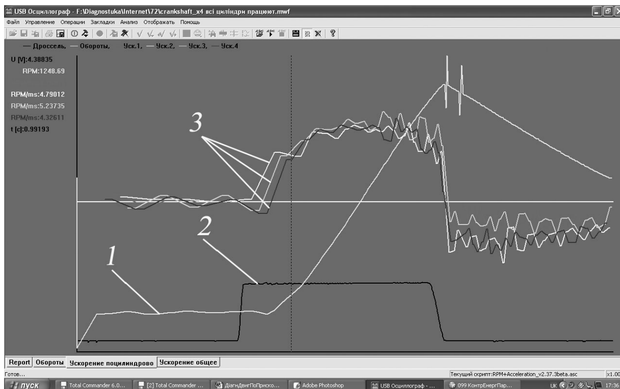
1 – сигнал частоти обертання колінчастого вала; 2 – сигнал відкриття дросельної заслінки; 3 – сигнали прискорень окремих циліндрів
