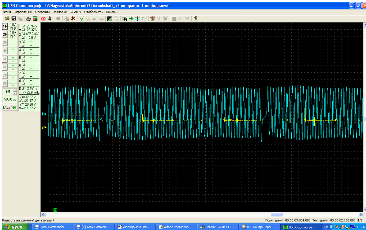
Рисунок 5 – Фрагмент осцилограми частоти обертання колінчастого вала двигуна з одним непрацюючим цилиндром
