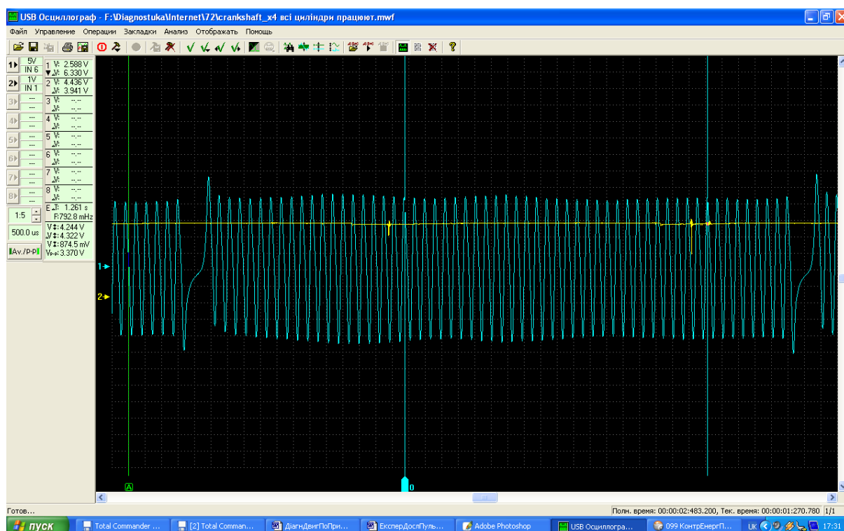
Рисунок 3 – Фрагмент осцилограми частоти обертання колінчастого вала справного двигуна
