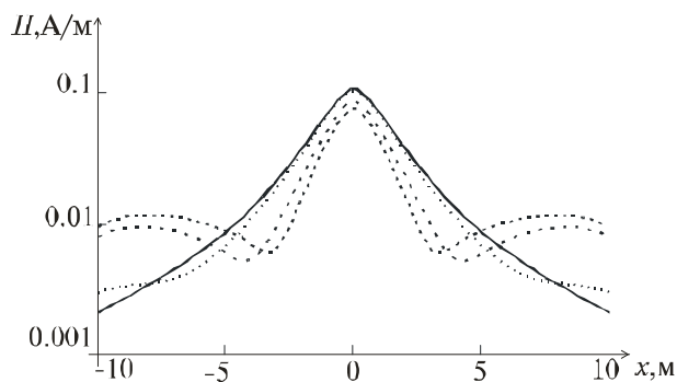
Рис. 7. Залежність горизонтальної складової напруженості магнітного поля від частоти
