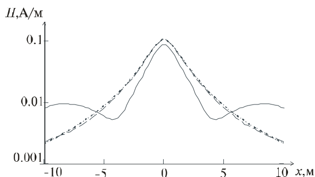
Рис. 8. Залежність горизонтальної складової напруженості магнітного поля від провідності ґрунту
