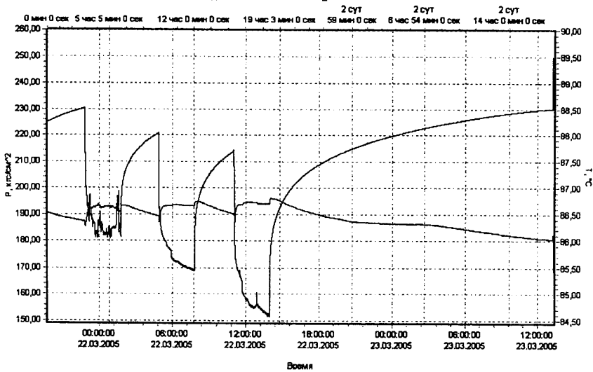
Рисунок 5 - Изменение забойного давления по 3-му прибору.
