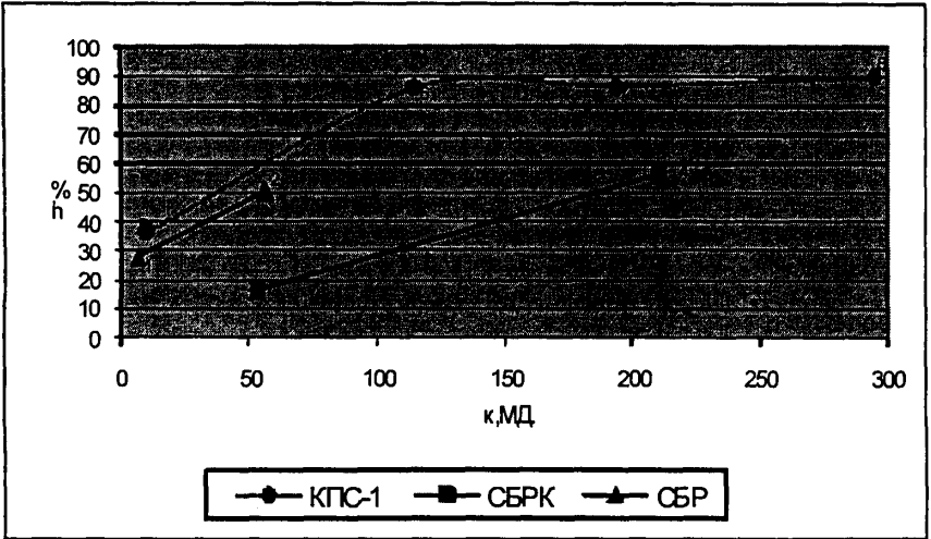
Рисунок 1- Влияние начальной проницаемости ядра на величину коэффициента восстановления проницаемости для различных технологических жидкостей.
