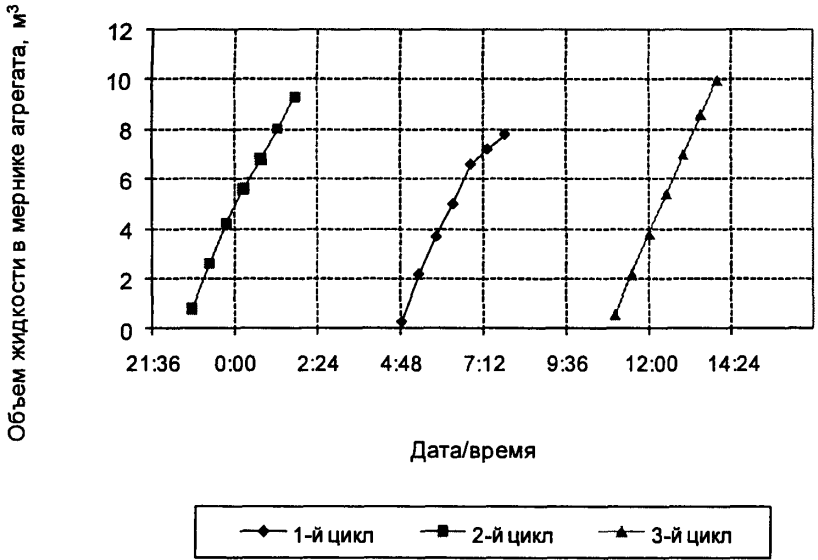
Рисунок 3 - Приток жидкости по трем циклам обработки.
