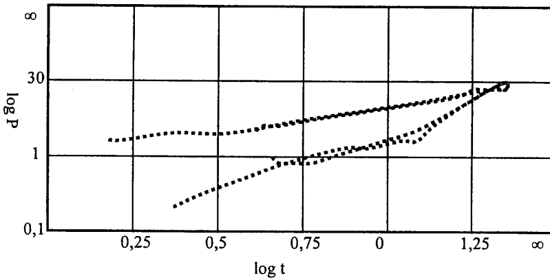
Рисунок 6 - КВД и ее производная в билогарифмических координатах.
