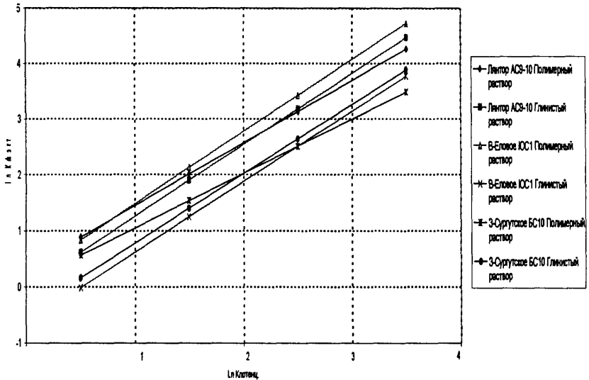
Рисунок 2 - Зависимость фактической продуктивности от потенциальной пластов ЮС 1 , БС 10 , АС 9-10 , вскрытых бурением с применением полимерного бурового раствора и глинистого на основе КМЦ
