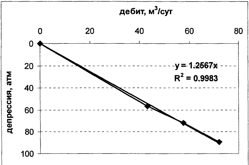
Рисунок 4 - Индикаторная диаграмма.
