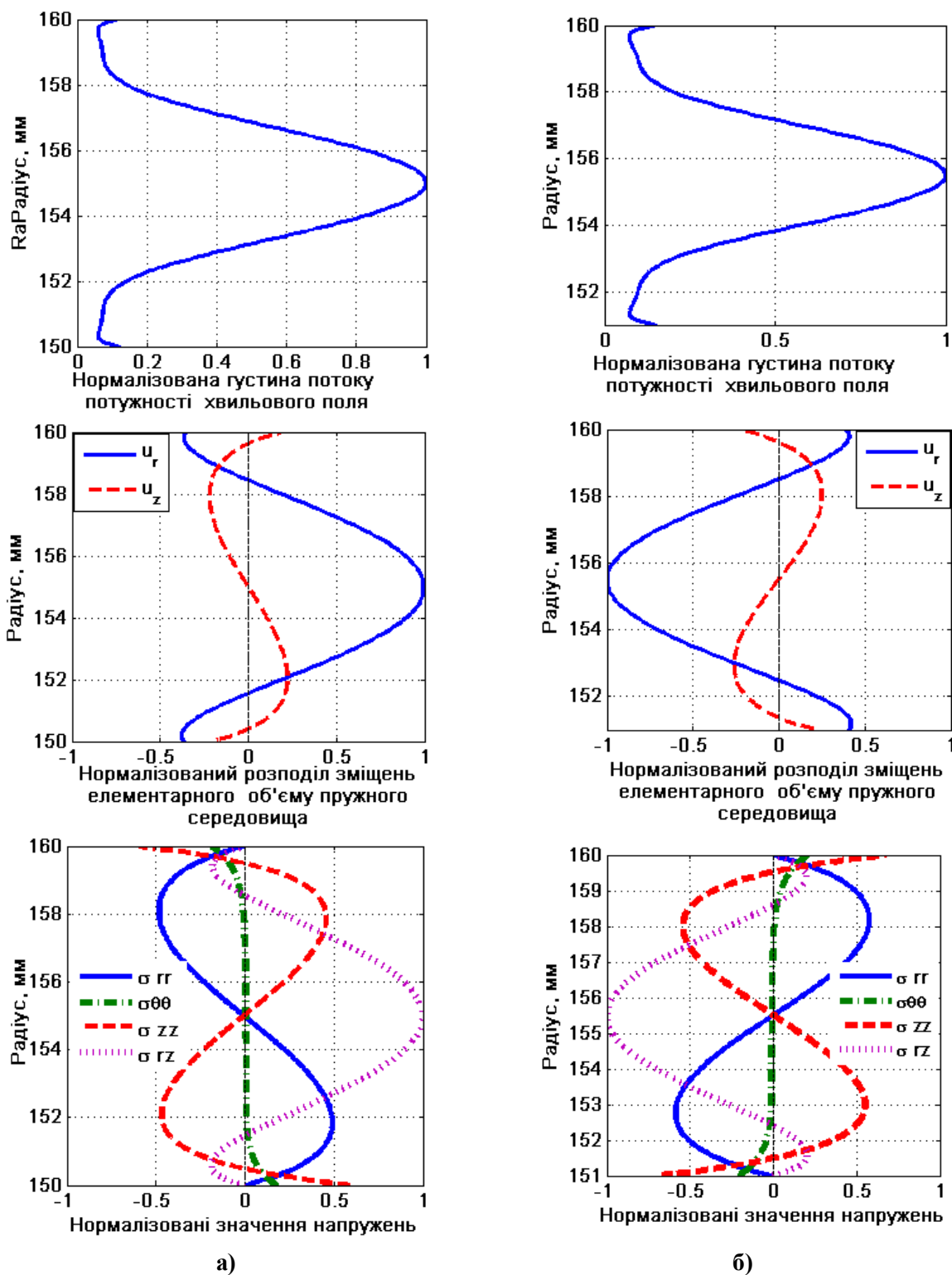
Рисунок 4 – Форми розподілу хвильового поля нульової поздовжньої моди УСХ по товщині стінки труби діаметром 320 мм за частоти спрямованої хвилі 1 МГц
