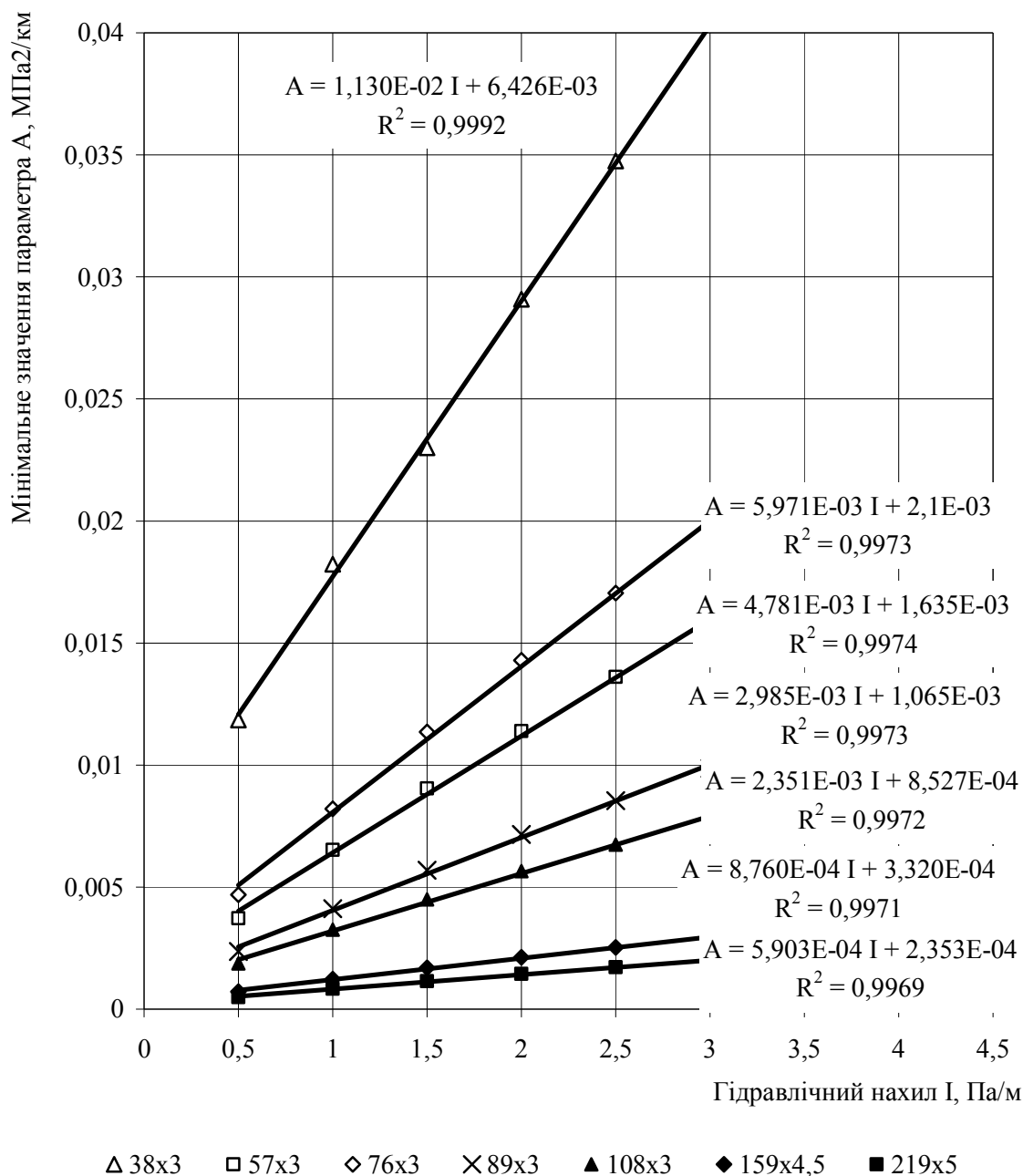
Рисунок 2 – Графічні залежності мінімального значення параметра A в поліетиленовій трубі середнього тиску від гідравлічного нахилу в сталевій трубі низького тиску за умови збереження пропускної здатності
