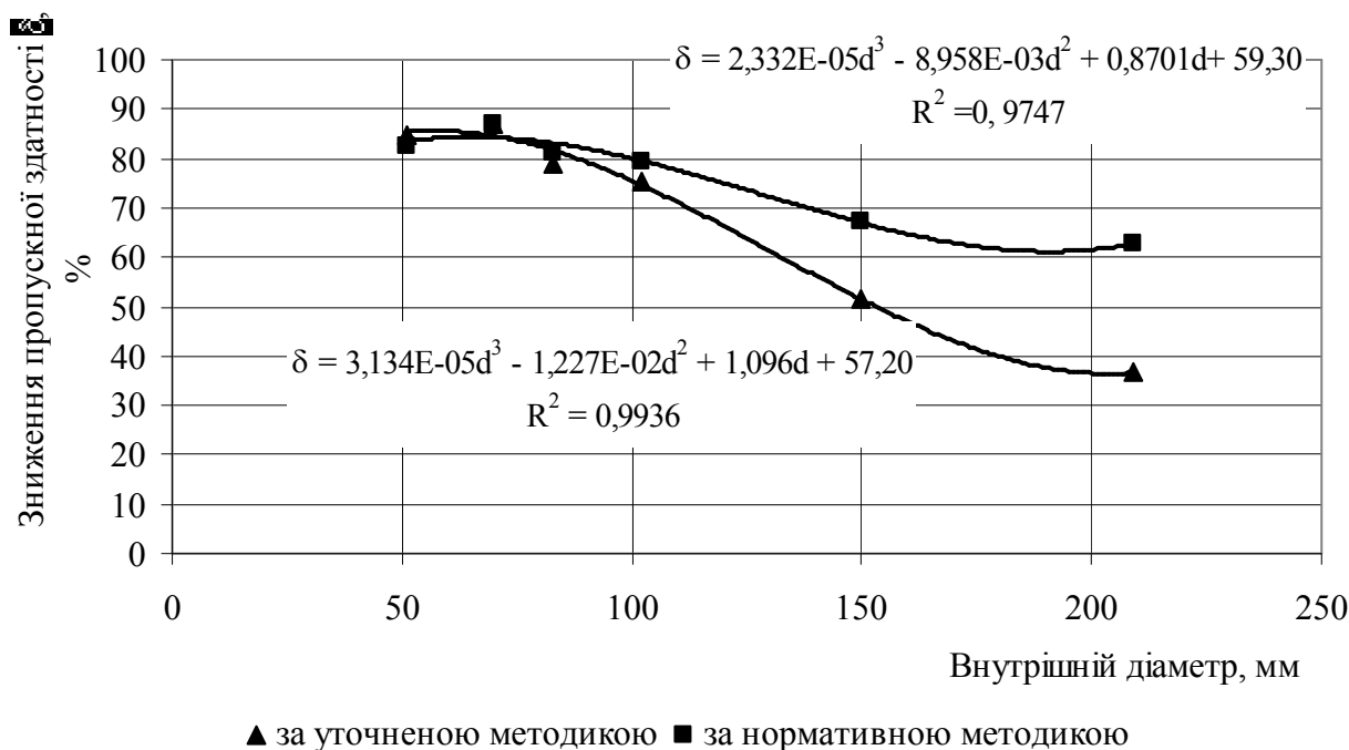
Рисунок 1 – Залежність зменшення пропускної здатності газопроводу від діаметра сталевих труб у разі її заміни на поліетиленову без зміни робочого тиску для гідравлічного нахилу 2 Па/м
