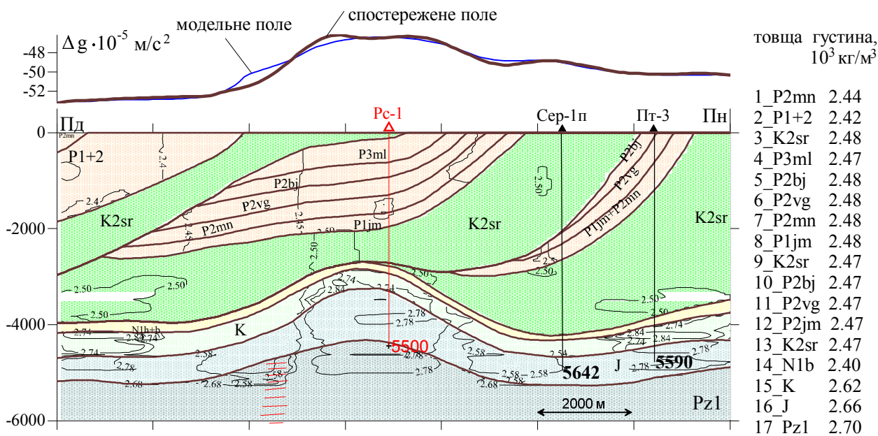
Рисунок 4 – Площа Руська. Геологічний профіль I-I (Склали Л.С. Мончак, С.Г. Анікєєв, В.П.Степанюк, 2009 р.)
