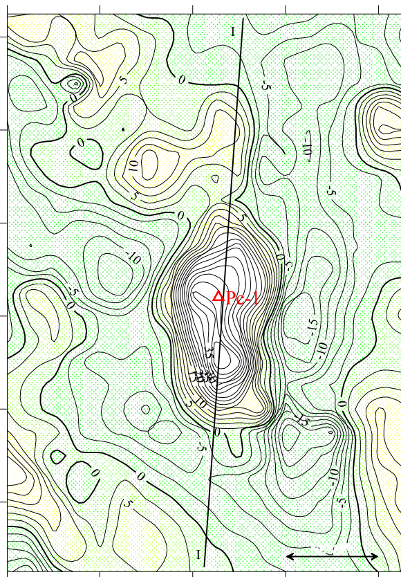
Рисунок 2 – Площа Руська. Локальні аномалії поля сили тяжіння для орієнтовної глибини простереження 0÷5000 м
