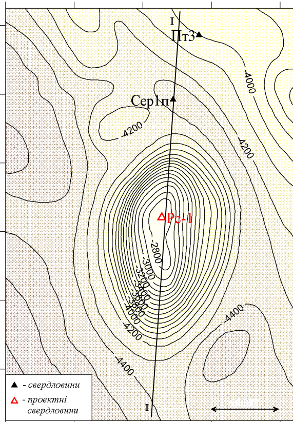
Рисунок 3 – Площа Руська. Структурна карта покрівлі мезозойських (крейдових) відкладів (Склав Л.С. Мончак, 2010 р.)
