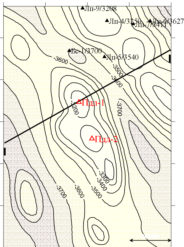
Рисунок 6 – Південнолопушнянська площа. Структурна карта покрівлі мезозойських відкладів (Склав Л.С. Мончак, 2010 р.)
