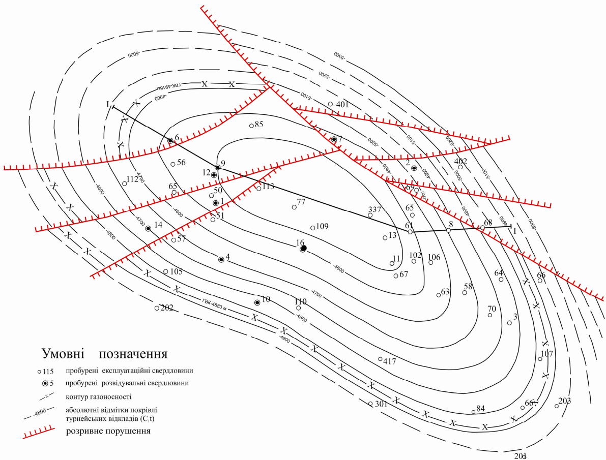
Рисунок 1 – Яблунівське нафтогазоконденсатне родовище . Структурна карта покрівлі турнейського горизонту (C 1t ) [11]
