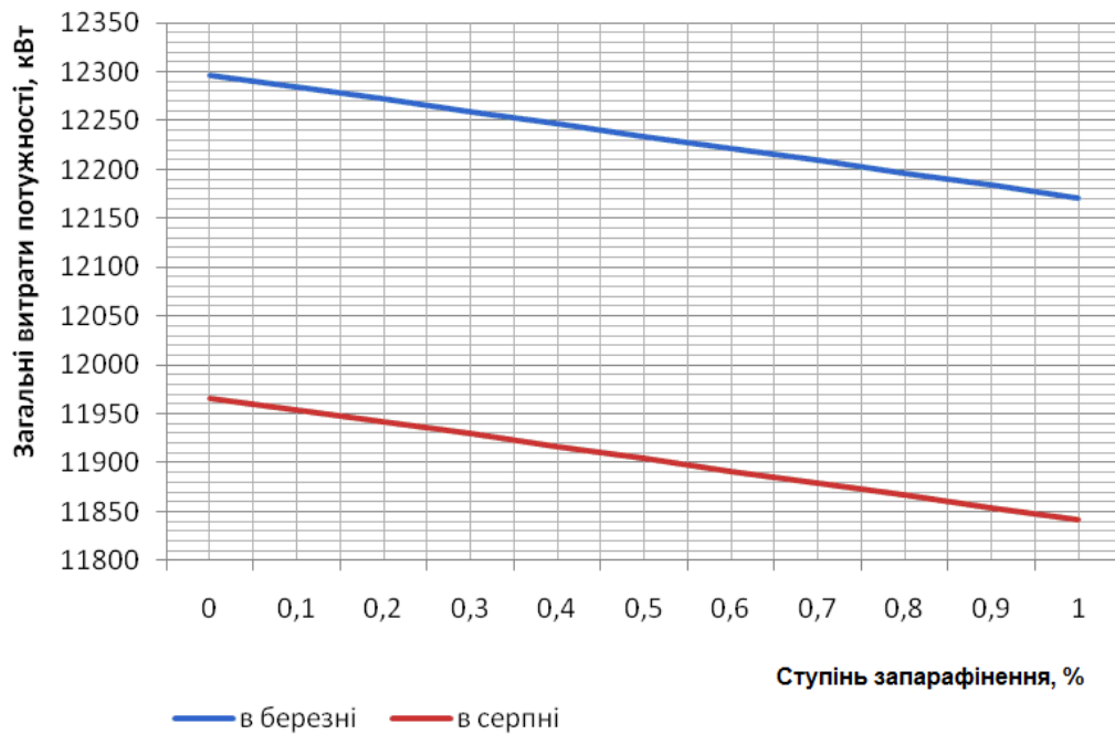
Рисунок 2 – Вплив запарафінення трубопроводу на загальні витрати потужності
