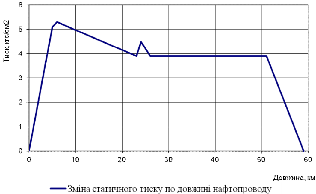
Рисунок 4 – Діаграма статичних тисків по довжині лінійної частини нафтопроводу Долина - Дрогобич
