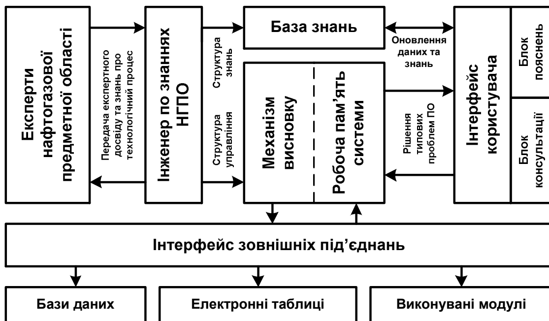
Рисунок 1 – Базові компоненти експертної системи
