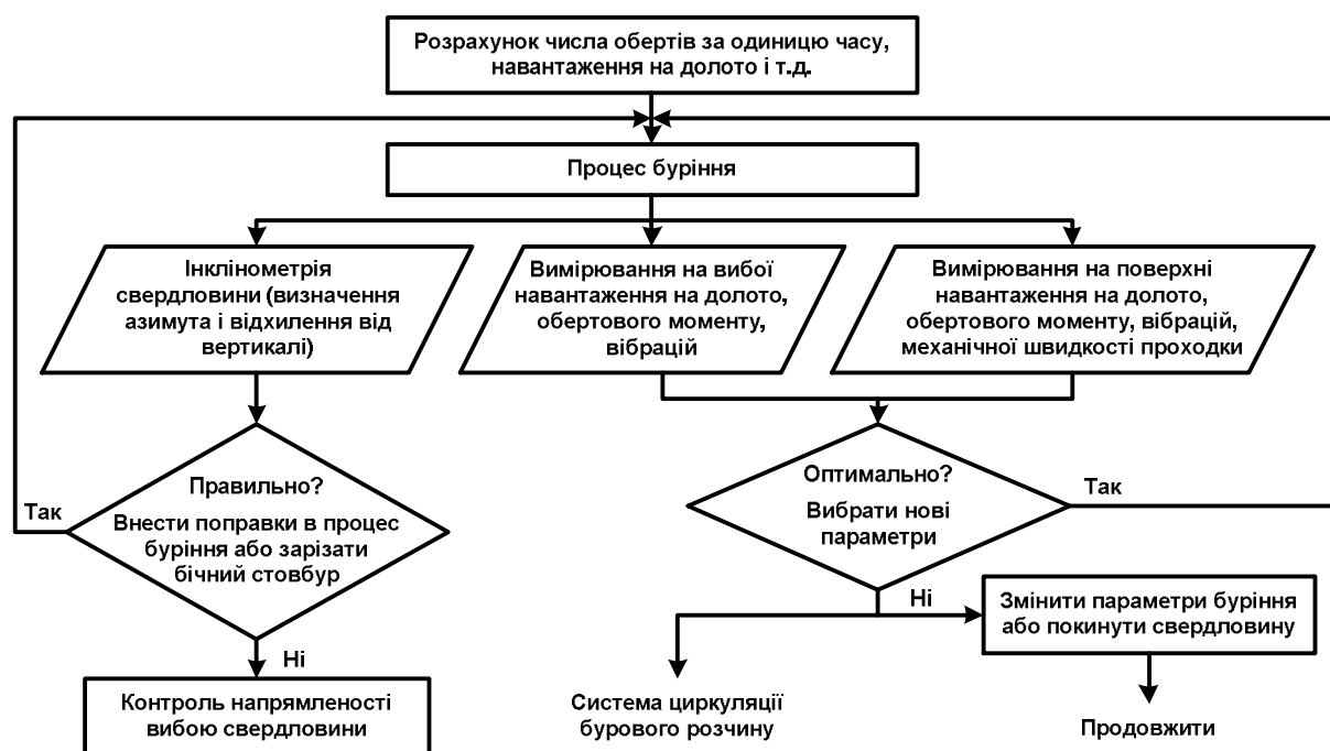
Рисунок 5 – Концептуальна структурна схема контролю долота на основі методів штучного інтелекту
