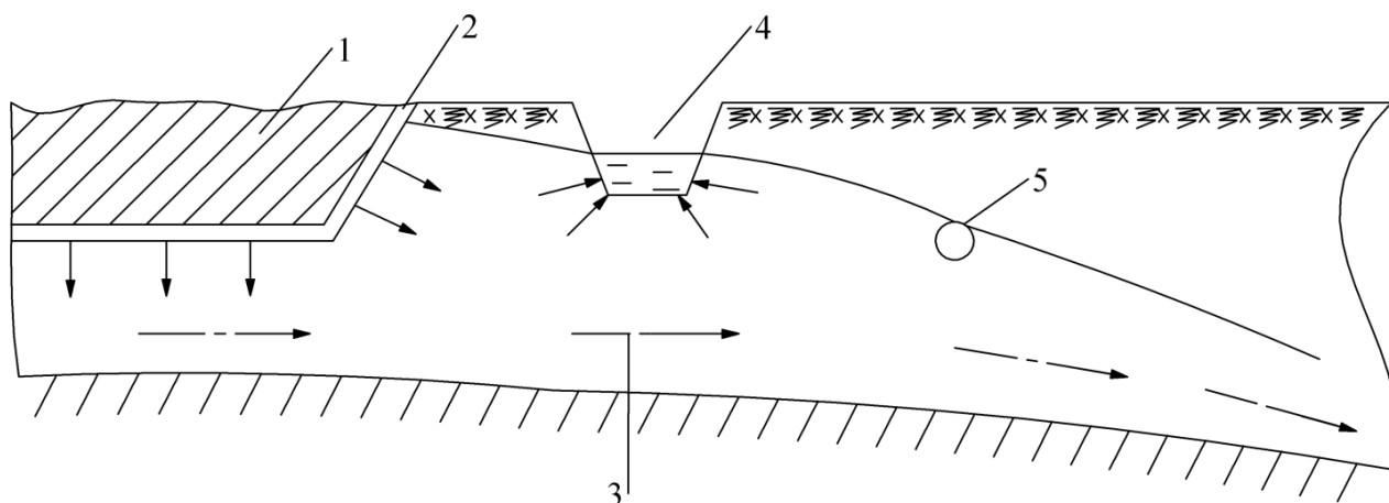
Рис.1. Схема перехоплення ґрунтового потоку ловчим каналом та дренажною лінією з масиву сміттєзвалища та прилеглої до нього території:
