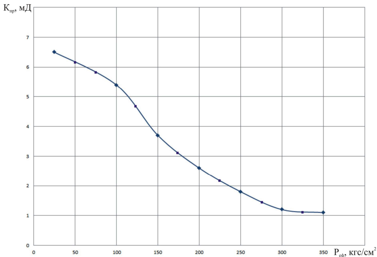
Рисунок 3 – Залежність абсолютної газопроникності від ефективного тиску
