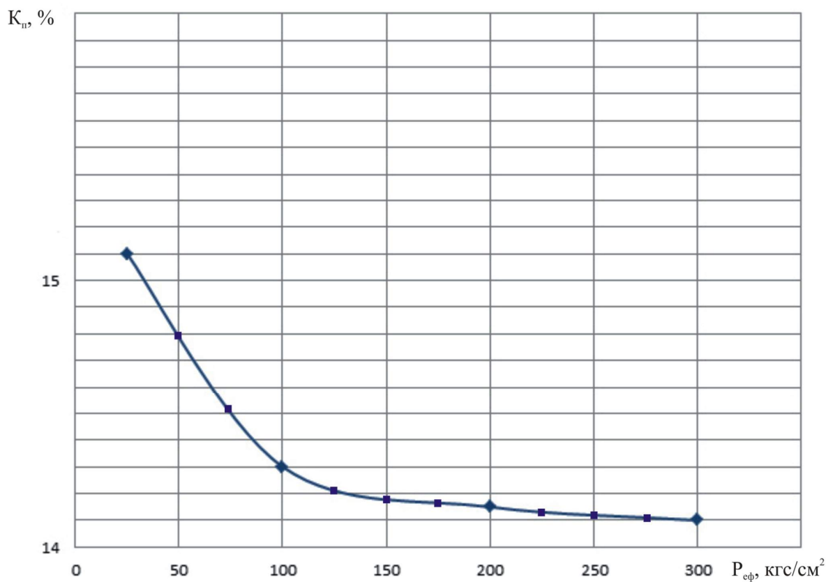
Рисунок 4 – Зміна відкритої пористості від ефективного тиску
