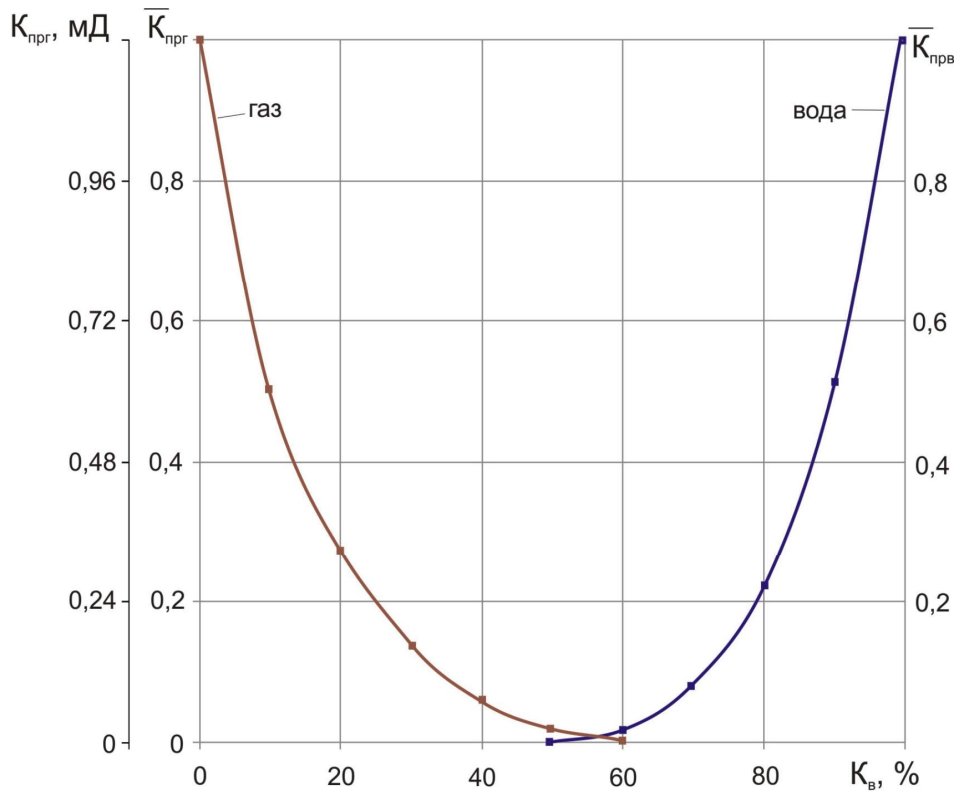
Рисунок 5 – Залежність фазових і відносних фазових проникностей для газу і води від водонасичення (проба № Ш-2, K_n=14,1 \% , K=51 \% )
