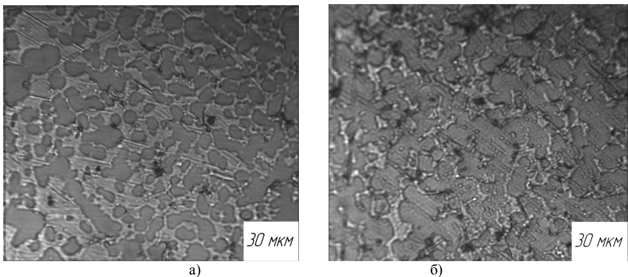
а) 15 хв; б) 45 хв
