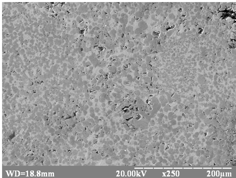
Рисунок 9 – Мікроструктура матеріалу \text{Cr}_3\text{C}_2 -марганцевий мельхіор
