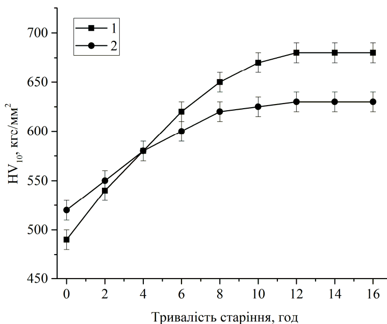
1 – тривалість просочування 15 хв.; 2 – тривалість просочування 45 хв. Рисунок 11 – Залежність твердості композитів від тривалості старіння
