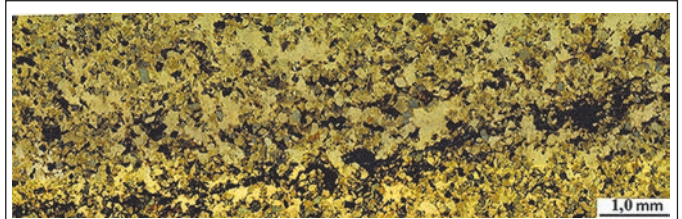
Рис. 2. Зразок GR-1. Панорамне зображення шліфа до соляно-кислотної обробки та взаємодії породи з сучасним піноутворюючим композитом. Показано фрагмент лінійно-розсіяної зони, збагаченої органічною речовиною, яка виповнює тріщини та каверни. В межах подібних зон властиве зростання кількості кальциту у складі цементу
