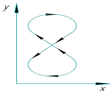
Рисунок 4 – Фігура Ліссажу
