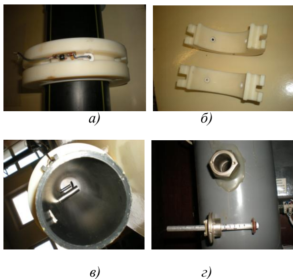
Рисунок 2 – Варіанти установки акустичних давачів на поверхні труби (а, б) та всередині труби (в, г) на прикладі труб лабораторної експериментальної установки
