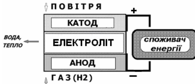
Рисунок 1 – Принципова схема будови паливної комірки
