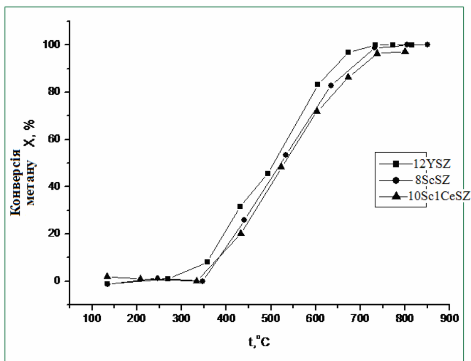
Рисунок 4 – Каталітична активність NiO-ZrO 2 у складі різних електролітів
