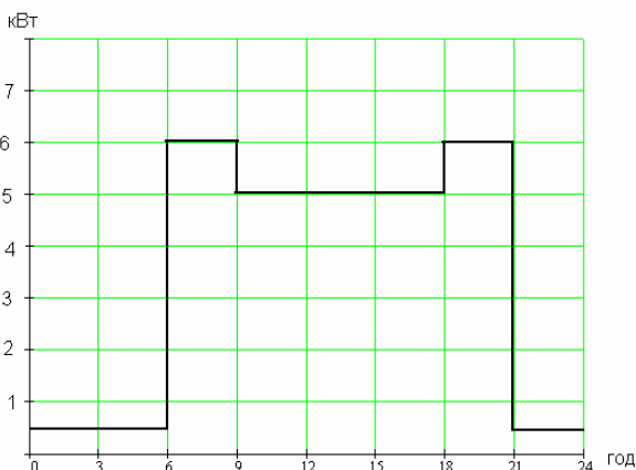
Рисунок 8 – Графік споживання потужності протягом доби
