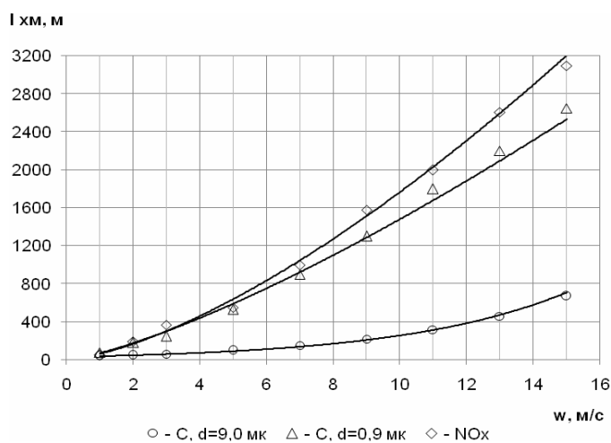
Рисунок 10 – Динаміка зміни зони впливу димової хмари на рівні приземного шару залежно від вітрової активності атмосферного повітря з урахуванням фізико-хімічних характеристик забруднюючих речовин
