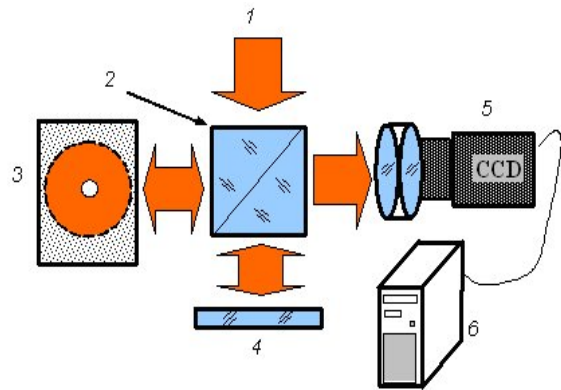
1 – розширений лазерний промінь; 2 – світлоподільник; 3 – зразок, що досліджувався; 4 – опорне дзеркало; 5 – відеокамера; 6 – ПК
