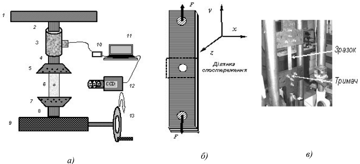
1 – нерухома плита; 2, 4, 8 – тяги; 3 – динамометр; 5, 7 – тримачі; 6 – зразок; 9 – редуктор з гвинтовим механізмом; 10 – індикаторний пристрій для контролю величини навантаження; 11 – комп'ютер; 12 – відеокамера; 13 – маховик ручного приводу
