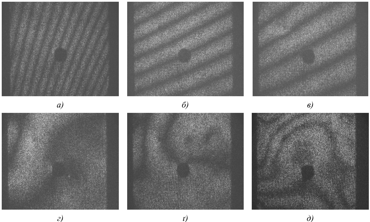
а) – 126 кгс; б) – 400 кгс; в) – 800 кгс; г) – 950 кгс; ґ) – 1100 кгс; д) – 1300 кгс
