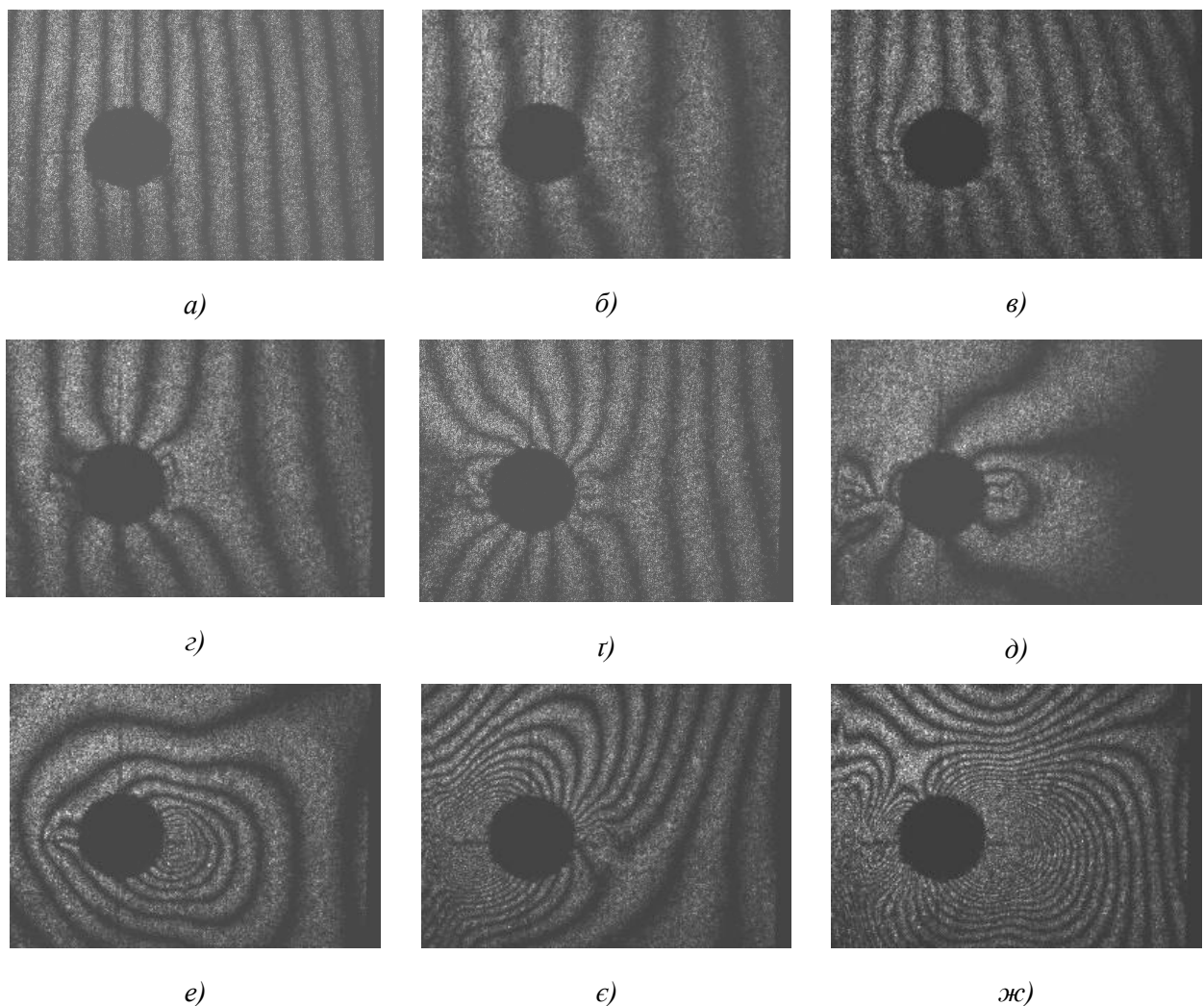
a) 400 кгс; б) 600кгс; в) 800 кгс; г) 1150 кгс; т) 1270 кгс, д) 1310 кгс, е) 1350 кгс; є) 1360 кгс; ж) 1160 кгс
