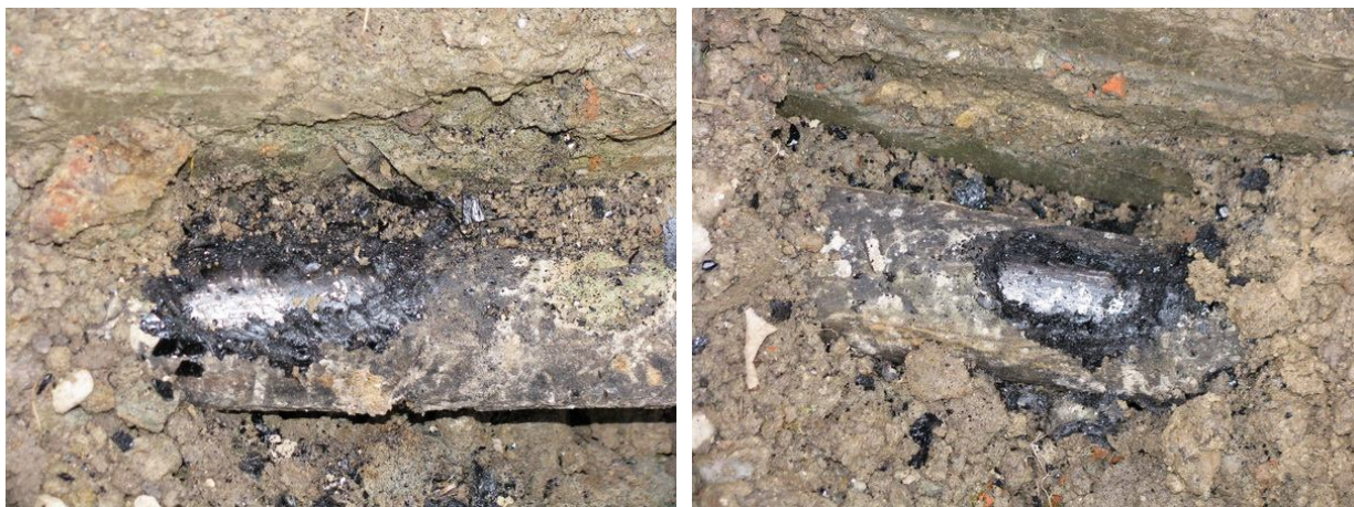
Рисунок 1 – Створені наскрізні дефекти ізоляційного покриття
