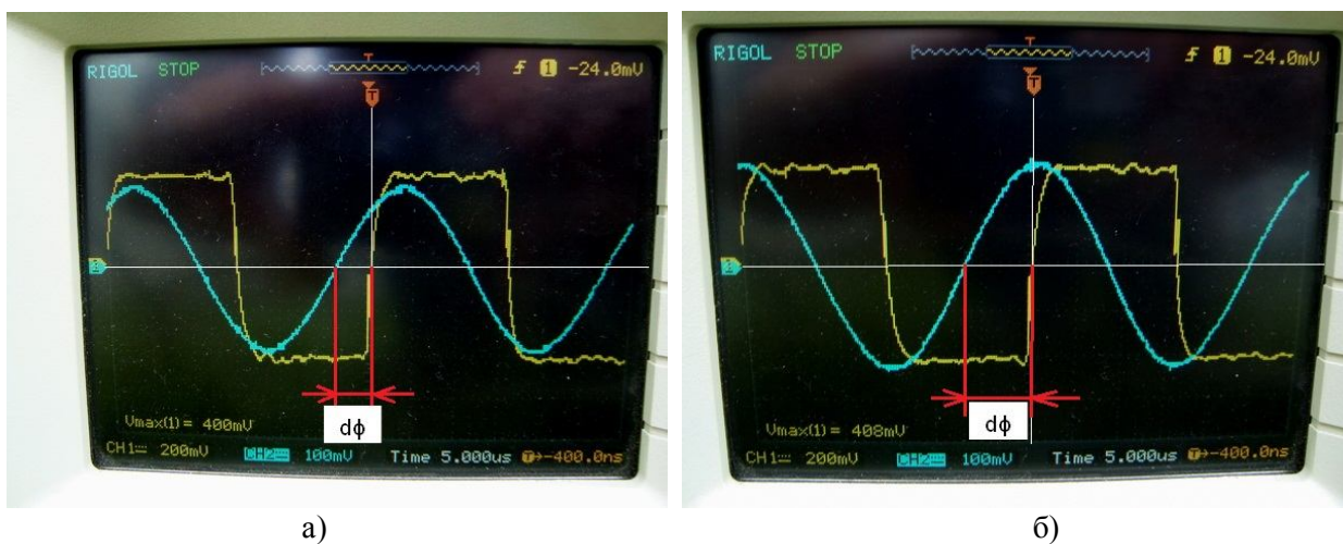
Рисунок 7 – Вимірювання зсуву фази за допомогою двоканального цифрового осцилографа: а) в точці L1 (рисунок 6); б) в точці L2 (рисунок 6)
