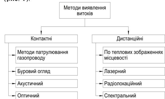
Рисунок 1 – Класифікація методів виявлення витоків газу з підземних газопроводів
