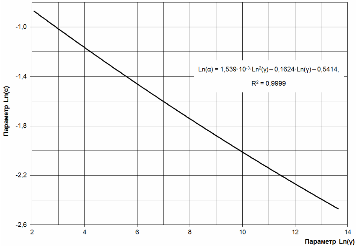
Рисунок 1 – Залежність величини відносного кута заповнення перерізу від коефіцієнта інтенсивності втрати енергії транспортованої рідини на самопливній ділянці ( \gamma \geq 8 )
