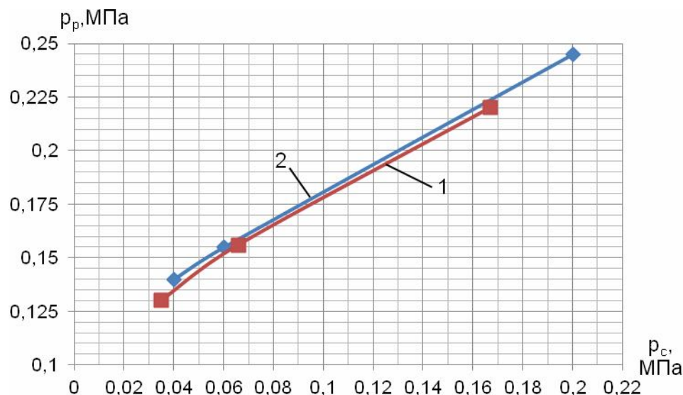
d_{кз}=12,5 мм, d_c = 6,6 мм; робочий потік – вода; 1 – інжектований потік вуглекислий газ; 2 – без інжектованого потоку
