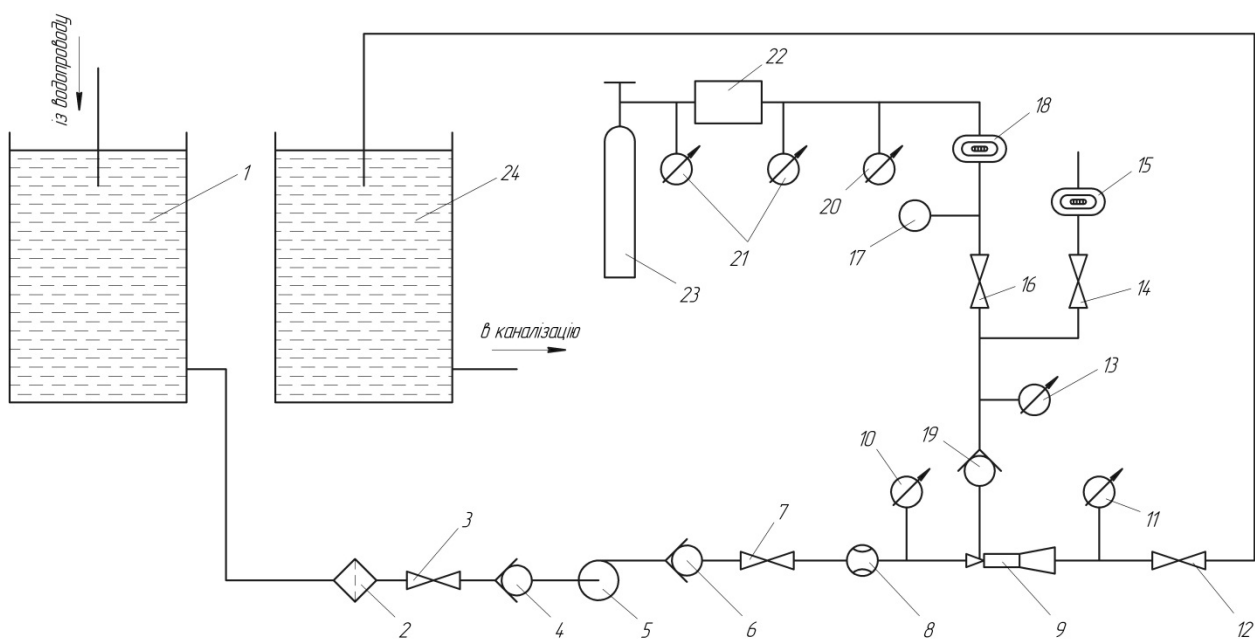
1 – резервуар води; 2 – фільтр насоса; 3, 7, 12, 14, 16 – крани; 4, 6, 19 – зворотні клапани; 5 – відцентровий насос JSWm15M; 8 – лічильник води GROSS MTK20; 9 – ежектор; 10, 11, 20 – манометри ДМ 05 – МП – ЗУ 100 – 0,6 МПа; 13 – мановакуумметр ДА 05160 – (-100 +500 кПа); 15 – газовий лічильник Арсенал GMSG6; 17 – термометр ТБ – 80 – 50 0+120 – 1,5; 18 – лічильник газу ротаційний G10 РЛ – ЕХ; 21 – манометр редуктора газового балона з CO 2 ; 22 – редуктор балона; 23 – газовий балон з CO 2 ; 24 – приймальний резервуар для води з CO 2
