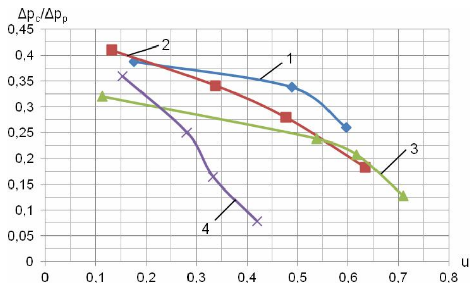
d_{кз}=10 мм: 1 – d_c = 5,4 мм ( f_3/f_{p1} = 3,43 ); 2 – d_c = 6,2 мм ( f_3/f_{p1} = 2,6 ); 3 – d_c = 5 мм ( f_3/f_{p1} = 4,0 ); 4 – d_c = 6,6 мм ( f_3/f_{p1} = 2,3 ) (кран 12 прикритий; інжектований потік – CO 2 )
