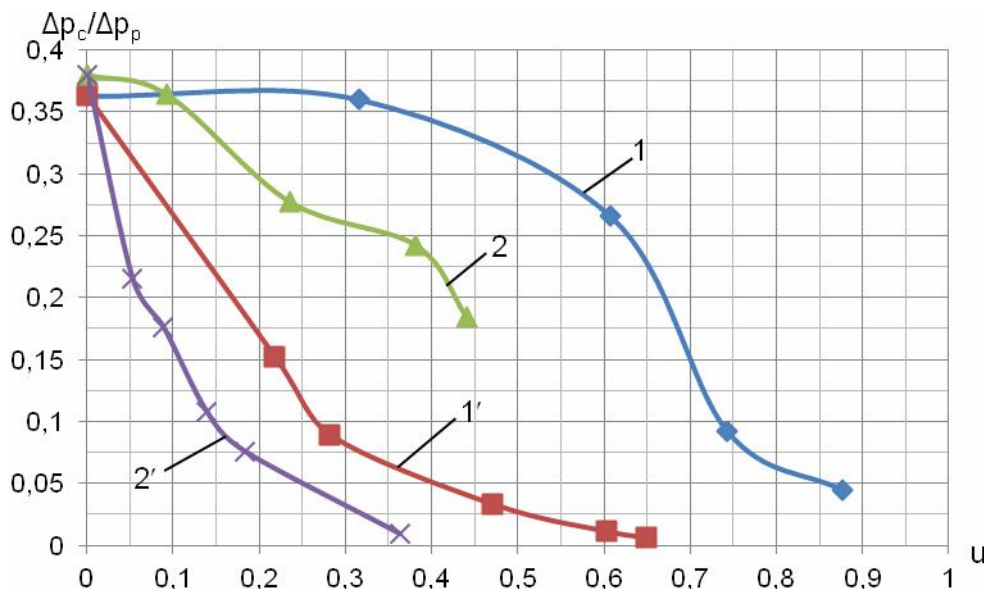
d_{кз}=10 мм: 1 – d_c = 5,4 мм ( f_3/f_{p1} = 3,43 ); 2 – d_c = 6,6 мм ( f_3/f_{p1} = 2,3 ) – інжектований потік вуглекислий газ; 1' – d_c = 5,4 мм ( f_3/f_{p1} = 3,43 ); 2' – d_c = 6,6 мм ( f_3/f_{p1} = 2,3 ) – інжектований потік повітря
