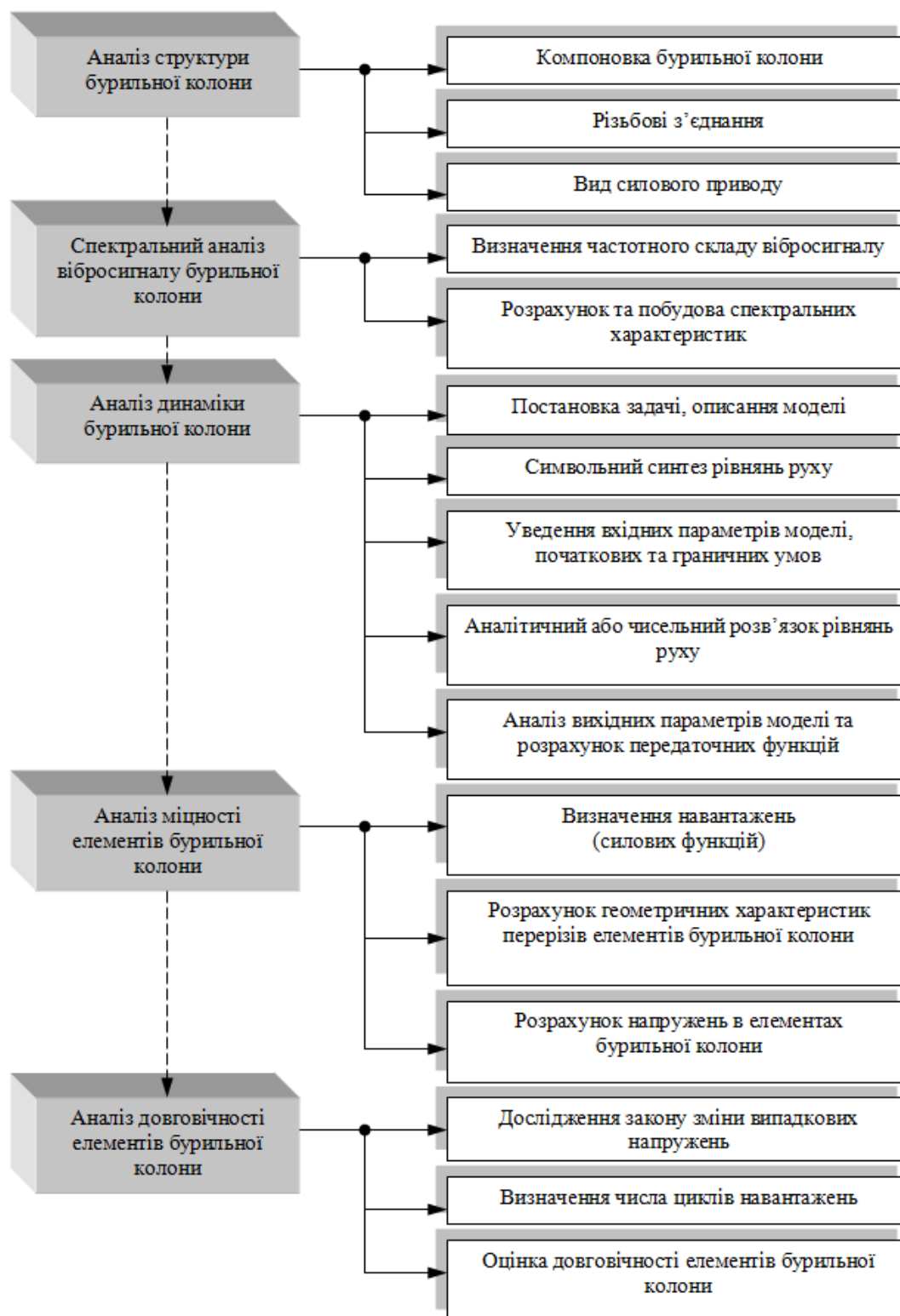
Рисунок 3 – Схема алгоритму для оцінки довговічності її елементів в умовах вібраційного навантаження
