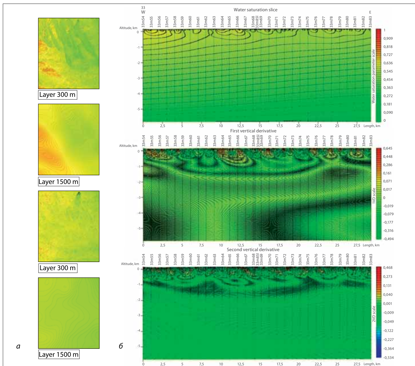
Рис. 2. Щільності потоку теплового випромінювання (а – верхні два фрагменти) та показник відносної водонасиченості (а – нижні два фрагменти) для глибин 300 і 1500 м. Вертикальні розрізи показника відносної водонасиченості (б) та відповідно зверху вниз його перша і друга похідні
