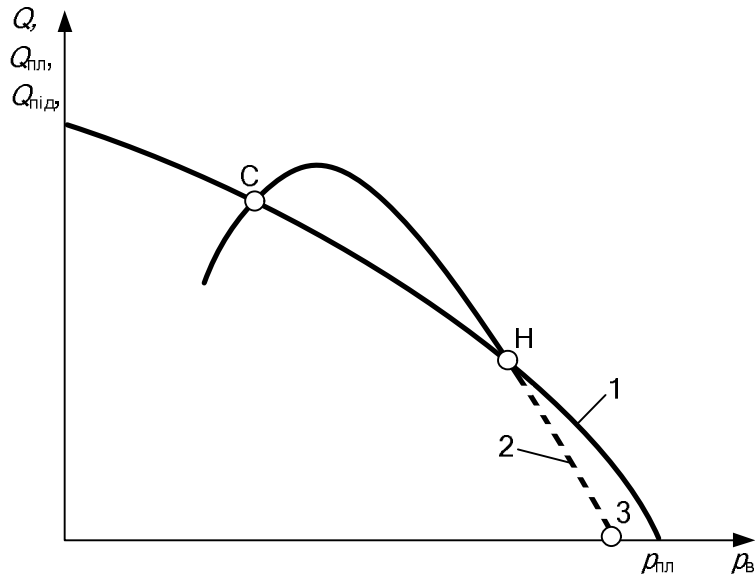
1 – індикаторна лінія Q_{пл}(p_в) ; 2 – модифікована крива ліфтування Q_{нід}(p_в) ; p_{пл} – пластовий тиск
