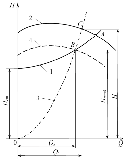
1 — сумарна характеристика трубопроводів; 2 — характеристика насоса для кількості обертів n_1 ; 3 — параболу подібних режимів роботи насоса; 4 — характеристика насоса після зменшення частоти обертання вала насоса до n_2 ; A — початкова робоча точка насосної установки; B — робоча точка після регулювання зміною частоти обертання; C — точка режиму роботи насоса з кількістю обертів n_1 подібного до режиму роботи трубопроводу з подачею Q_3 і напором H_{необ}
