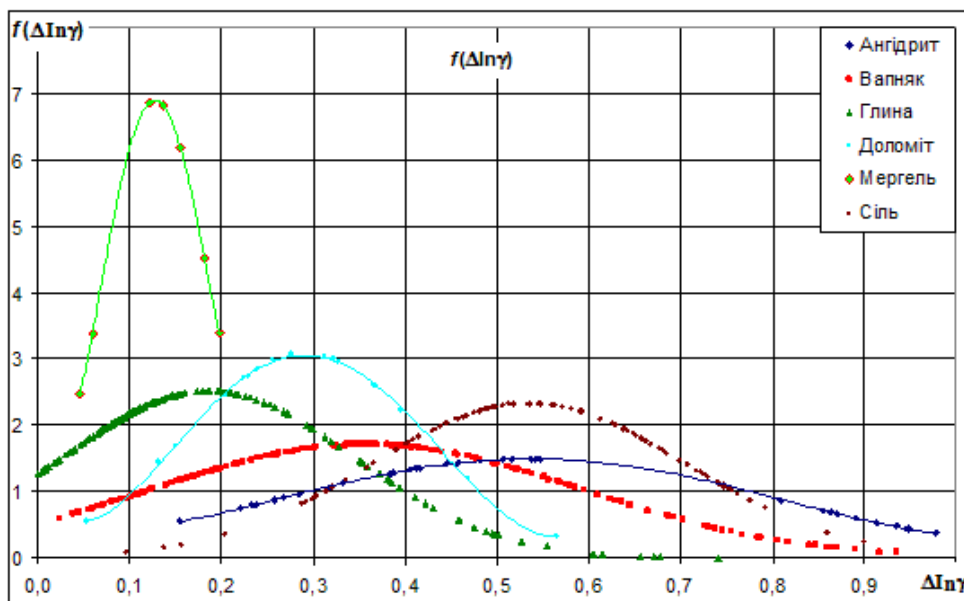
Рисунок 3 – Диференційні криві, що описують фактичні розподіли ймовірності значень подвійного різницевого параметра \Delta In\gamma для певних літологічних міжсоляної карбонатно-хемогенної товщі
