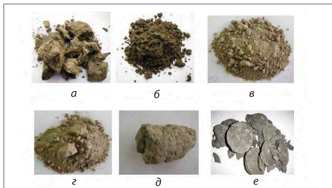
Рис. 2. Проби досліджуваного кернавого матеріалу: а – керна 1 (496 м); б – керна 1 (492,5 м); в – керна 2 (475 м); г – керна 2 (473 м); д – керна 4 (522 м); е – керна 6 (540 м)
