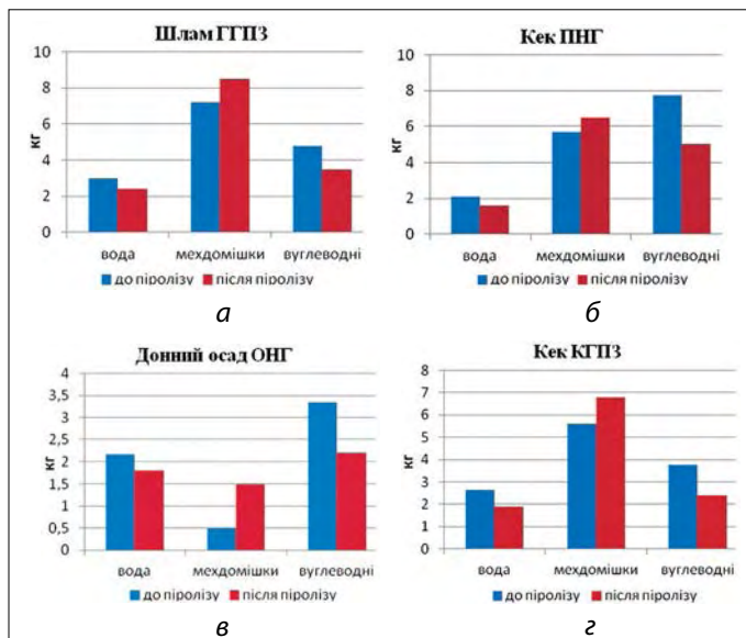
Рис. 4. Матеріальний баланс піролізу нафтошламів із NORM: а – шлам Гнідинцівського ГПЗ; б – кек НГВУ «Полтаванафтогаз»; в – донний осад з шламонакопичувача НГВУ «Охтирканафтогаз»; г – кек Качанівського ГПЗ
