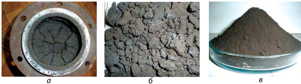
Рис. 6. Твердий продукт піролізу (напівкокс): а – у дослідній установці; б – вивантажений; в – подрібнений
