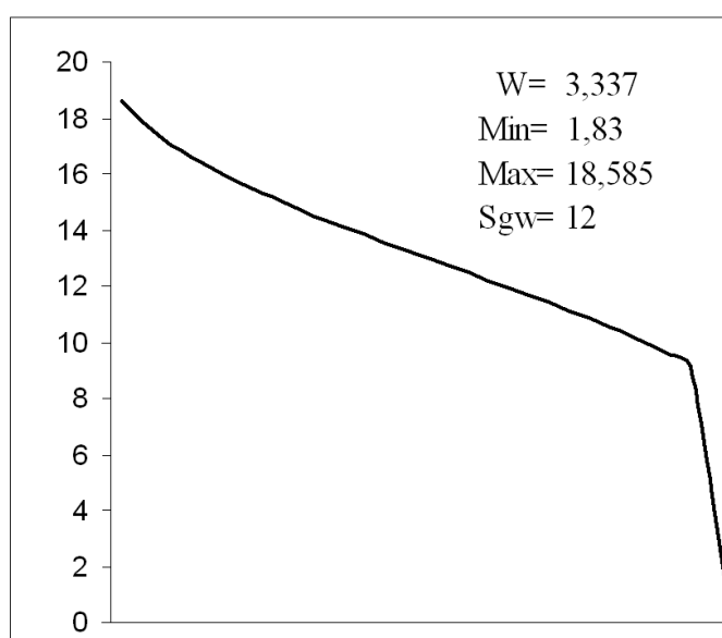
Рисунок 3 – Варіаційний ряд блоку навантаження при опусканні БК (L=1570 м)
