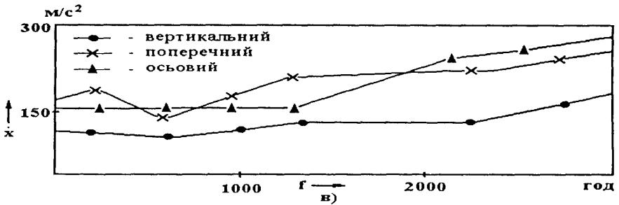
Рис. 1 – параметри вібрації двигуна ГТН-25 ГПА-25/76 (а – спектри вібрації; б, в – відповідно, залежності рівня вібрації у діапазоні 0-300Гц і 0-10кГц від напрацювання).
