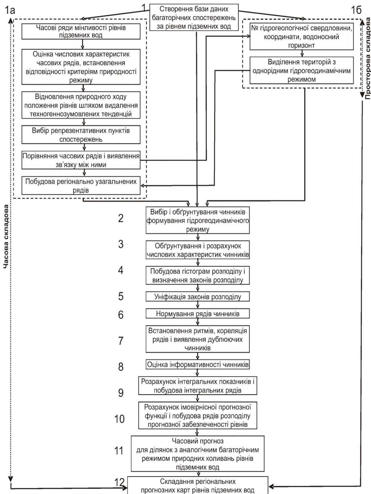
Рисунок 1 – Алгоритм дослідження і прогнозування багаторічних закономірностей природного гідрогеодинамічного режиму
