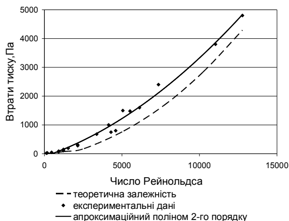
Рисунок 4 – Залежність втрат тиску на резиновому гнучкому шлангу від числа Рейнольдса
