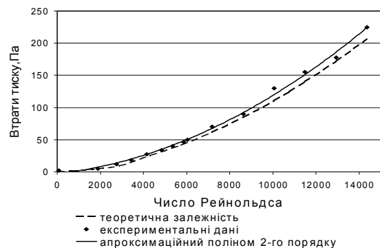
Рисунок 2 – Залежність втрат тиску на тертя в трубі від числа Рейнольдса на прямо-лінійній ділянці труби (з розрахунку на 1м)
