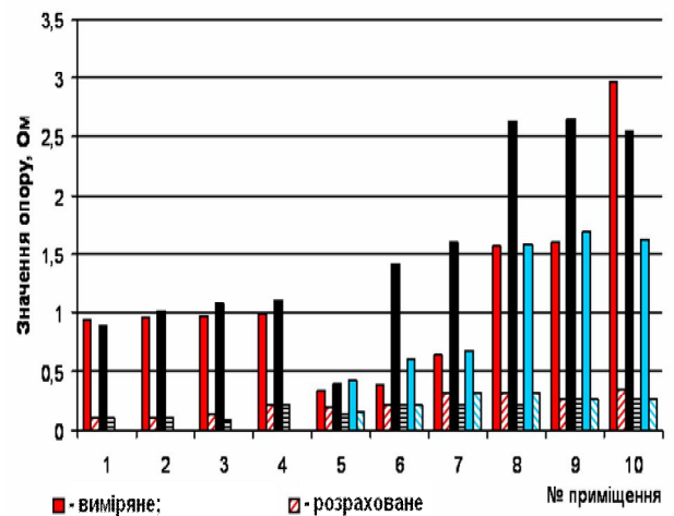
Рисунок 1 – Значення вимірних і розрахованих опорів ДЕНН
