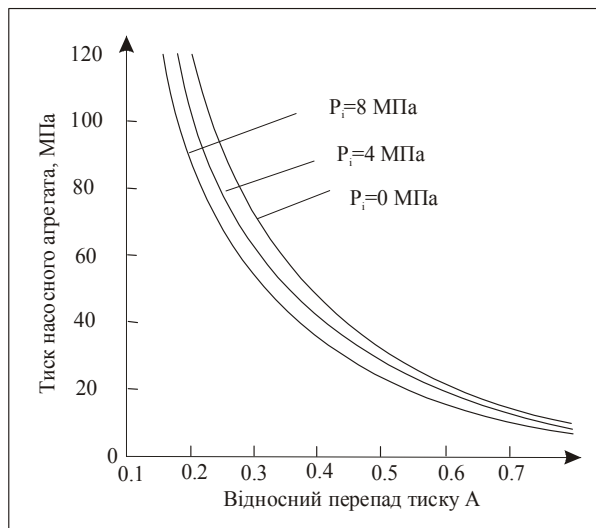
Рисунок .5 – Залежність тиску насосного агрегату від відносного перепаду тиску A за L=3000 м, P_n=0,4,8 МПа, Q_p=4,73 \cdot 10^{-3} м 3 /с, Q=40 м 3 /добу
