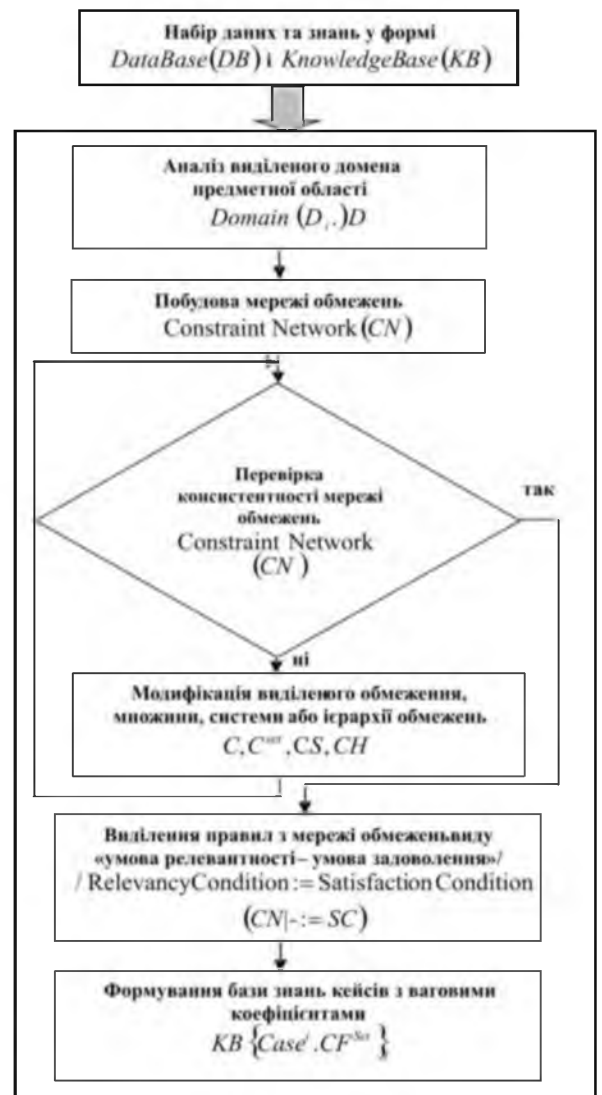
Рисунок 3 – Локалізація процедури побудови БЗ кейсів
